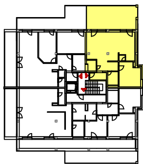
Pôdorys poschodia
