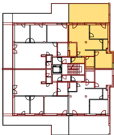
Pôdorys poschodia
